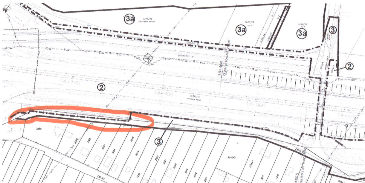
1. ábra Új M3 autópálya csomópont (19+130,54 km sz.) I. szakasz Kiviteli terv
